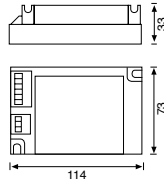
JK218 2x18W Elektronik Balast 5,00 USD 100 Ad. 114x73x33
